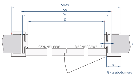
drzwi dwuskrzydłowe
