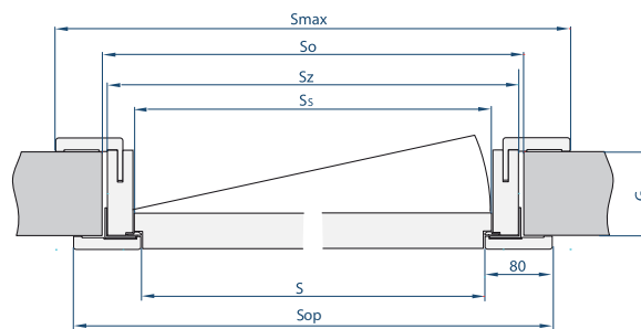
drzwi jednoskrzydłowe PRAWIE
