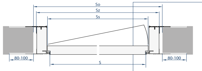
drzwi jednoskrzydłowe PRAWO
